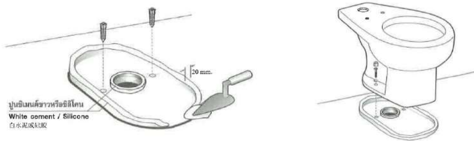
รูปที่ 4.54 ตัวอย่างก่อนแนบปูนซีเมนต์ขาว ตามแนวฐานของโถส้วม
