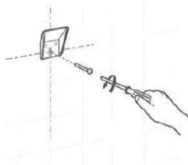
รูปที่ 4.75 ตัวอย่าง การติดตั้งโป๊สสาวะชาย แบบชนิดท่อน้ำทิ้งแยก
