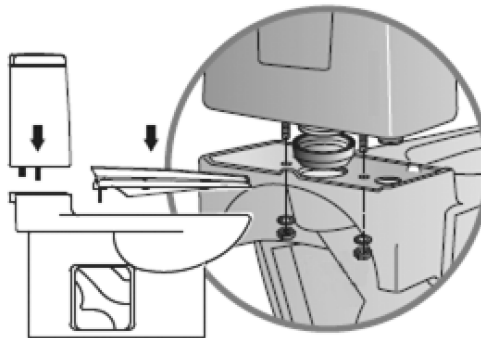
รูปที่ 4.39 ตัวอย่างการประกอบถังชักน้ำ และฝารองนั่งเข้ากับโถส้วม
