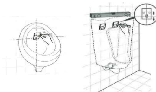
รูปที่ 4.82 ตัวอย่าง การติดตั้งโป๊สสาวะชาย แบบชนิดท่อน้ำทิ้งในตัว
