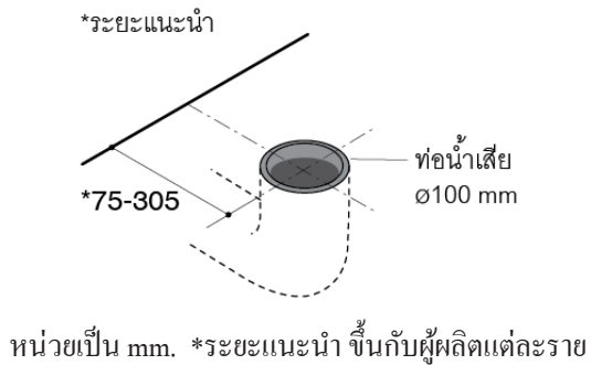
รูปที่ 4.34 ตัวอย่าง ระยะการติดตั้ง
