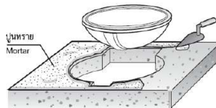
รูปที่ 4.69 ตัวอย่าง การติดตั้งอ่างล้างหน้า แบบฝังใต้เคาน์เตอร์
