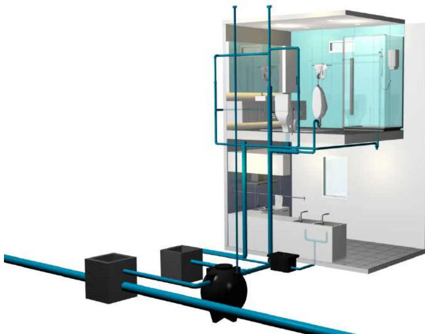
รูปที่ 4.94 แสดงระบบระบายน้ำภายในบ้านพักอาศัยและอุปกรณ์ต่าง ๆ (ที่มา : ท่อเอสซีจี)
