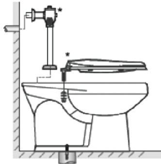
รูปที่ 4.52 ตัวอย่างการประกอบอุปกรณ์วาล์วขันล่างและฝารองนั่งเข้าโถส้วม
