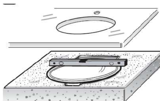
รูปที่ 4.71 ตัวอย่าง การติดตั้งอ่างล้างหน้า แบบวางบนเคาน์เตอร์
