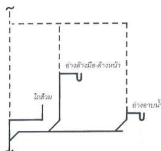
รูปที่ 1.6 รูปแผนผังแสดงการเดินท่อของระบบระบายน้ำสุขาภิบาลและระบบระบายอากาศในห้องน้ำ
