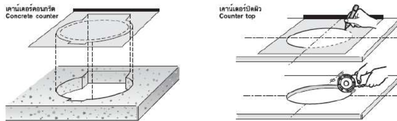
รูปที่ 4.68 ตัวอย่าง การติดตั้งอ่างล้างหน้า แบบฝังใต้เคาน์เตอร์
